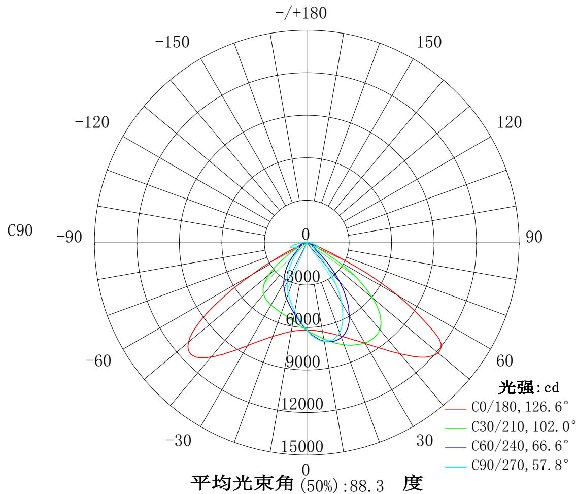
子午面配光曲线
