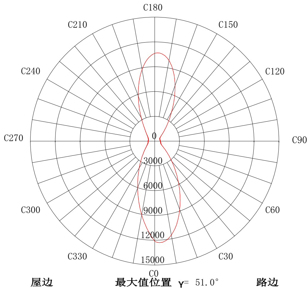
最大光强处圆锥面光强分布曲线
